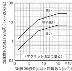
加速度—転がり軸受判定グラフ
