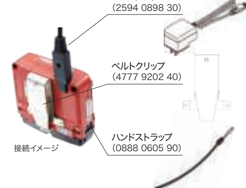
ACアダプター (2594 0898 30)
