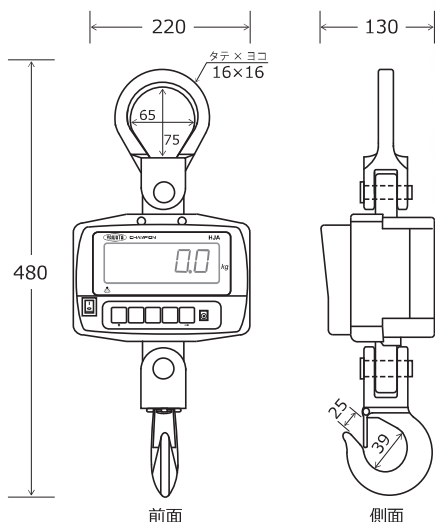
外形寸法図 単位 mm
