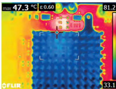
電子基板の温度分布を測定することで温度監視デバイスの適切な配置を決定できる
