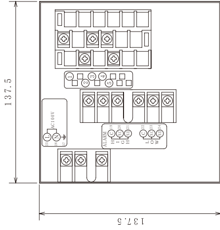
端子台図
