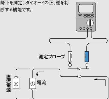
c) ダイオードテスト方法
