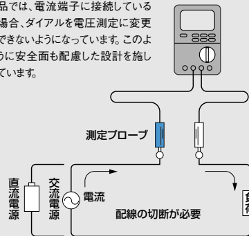
b) 電流の測定方法
