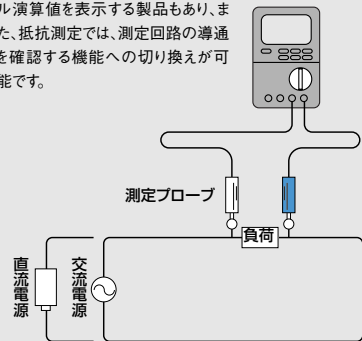
a) 電圧、抵抗の測定方法
