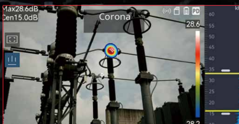
部分放電を識別(コロナ/浮遊/表面/粒子) 深深度も表示
