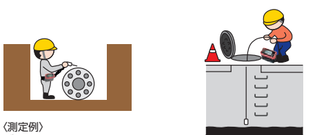
〈測定例〉 地下タンク内濃度測定
